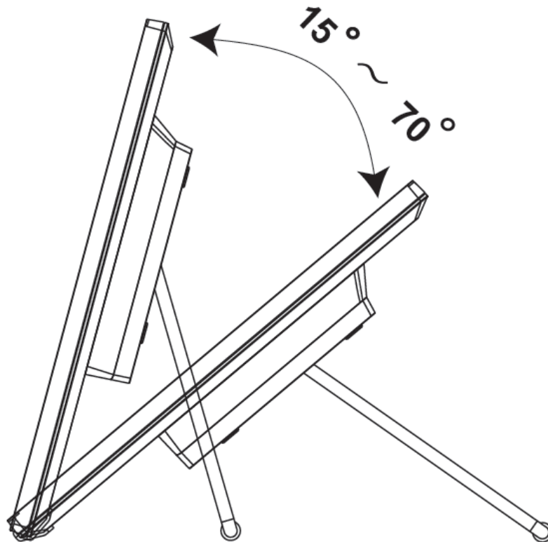
ABBILDUNG 3. MONITORWINKEL
