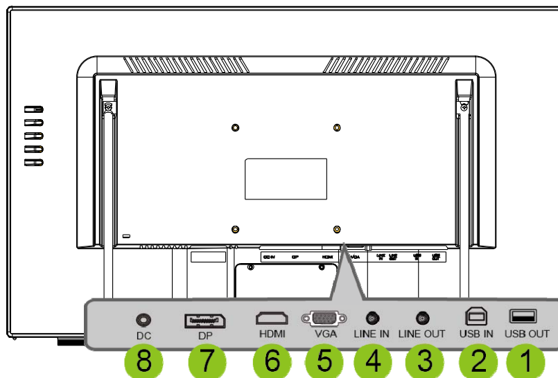
ABBILDUNG 2. ANSCHLISSEN AN EINEN PC
